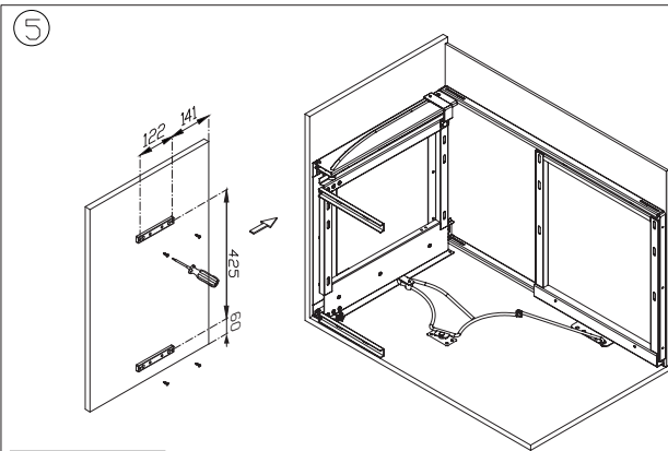
M4x25 SV/4
